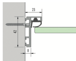
Profilé de dormant, raccord au mur
