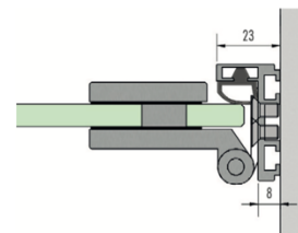
Profilé de dormant paumelle, raccord au mur
